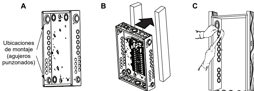
Fig 3: Montaje a ras
