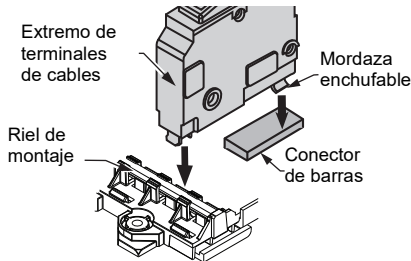
Fig 5: Interruptor automático QO en tándem
