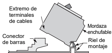
Fig 6: Interruptor automático Homeline estándar
