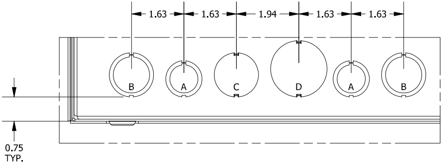
DETAIL B (3 PL.) (K.O. PATTERN)
