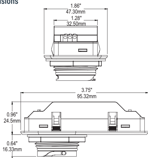
FSP-212 Dimensions
