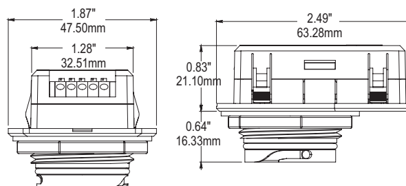
FSP-202 Dimensions
