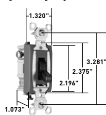
15 &amp; 20 Amp Lighted &amp; Pilot Lighted*
